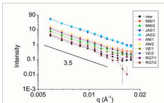
5. ábra Orgonasípok I=f(Q) görbéi
