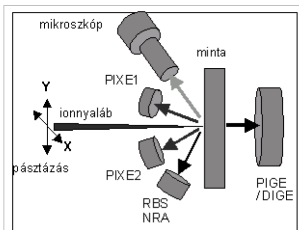
2. ábra. IBA mérési elrendezés kisenergiás PIXE (PIXE1: elemek a bórtól kezdődően), nagyenergiás PIXE (PIXE2: elemek a szilíciumtól kezdődően), részecske- (RBS, NRA), valamint gamma-detektorokkal. A nyaláb általában kollimálható, pásztázó nukleáris mikroszkópokban fókuszálható és a minta felületén X-Y irányokban számítógéppel vezérelten mozgatható (pásztázás). A mikroszkóp a minta és a nyalábfolt vizuális megfigyelésére szolgál (ld. http://www.atomki.hu/atomki/VdG/iba.html )
