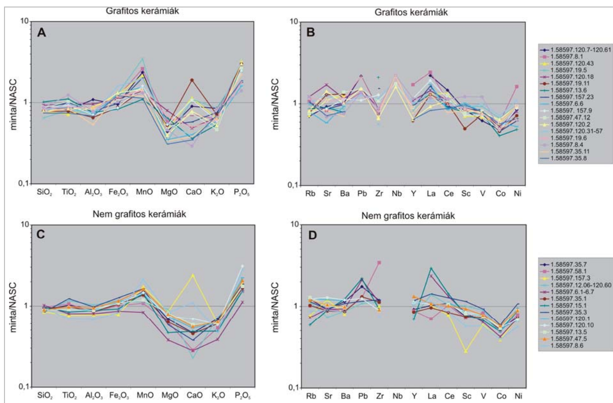
4. ábra Grafitos és nem grafitos kerámiák NASC-ra normált sokelemes gyakorisági diagramjai: A, C: főelemek, B, D: nyomelemek
