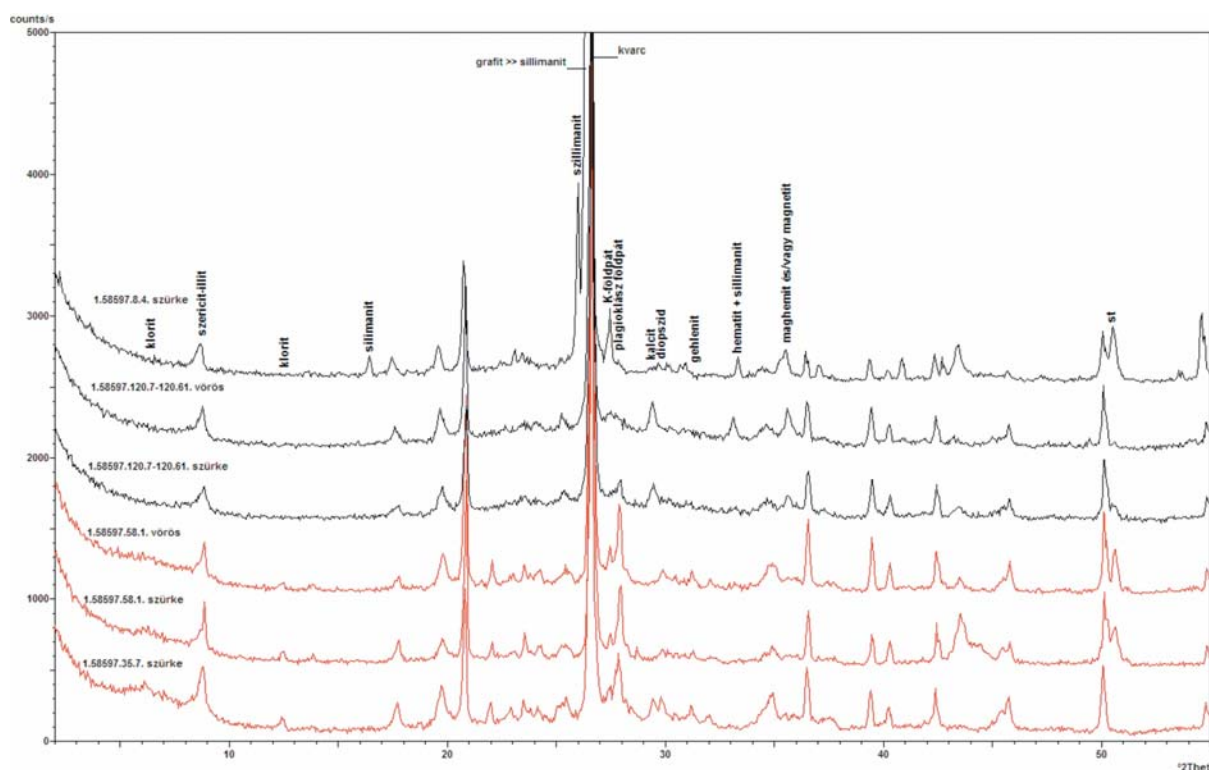
6. ábra Grafitos és nem grafitos kerámiák röntgen-diffraktogramjai
