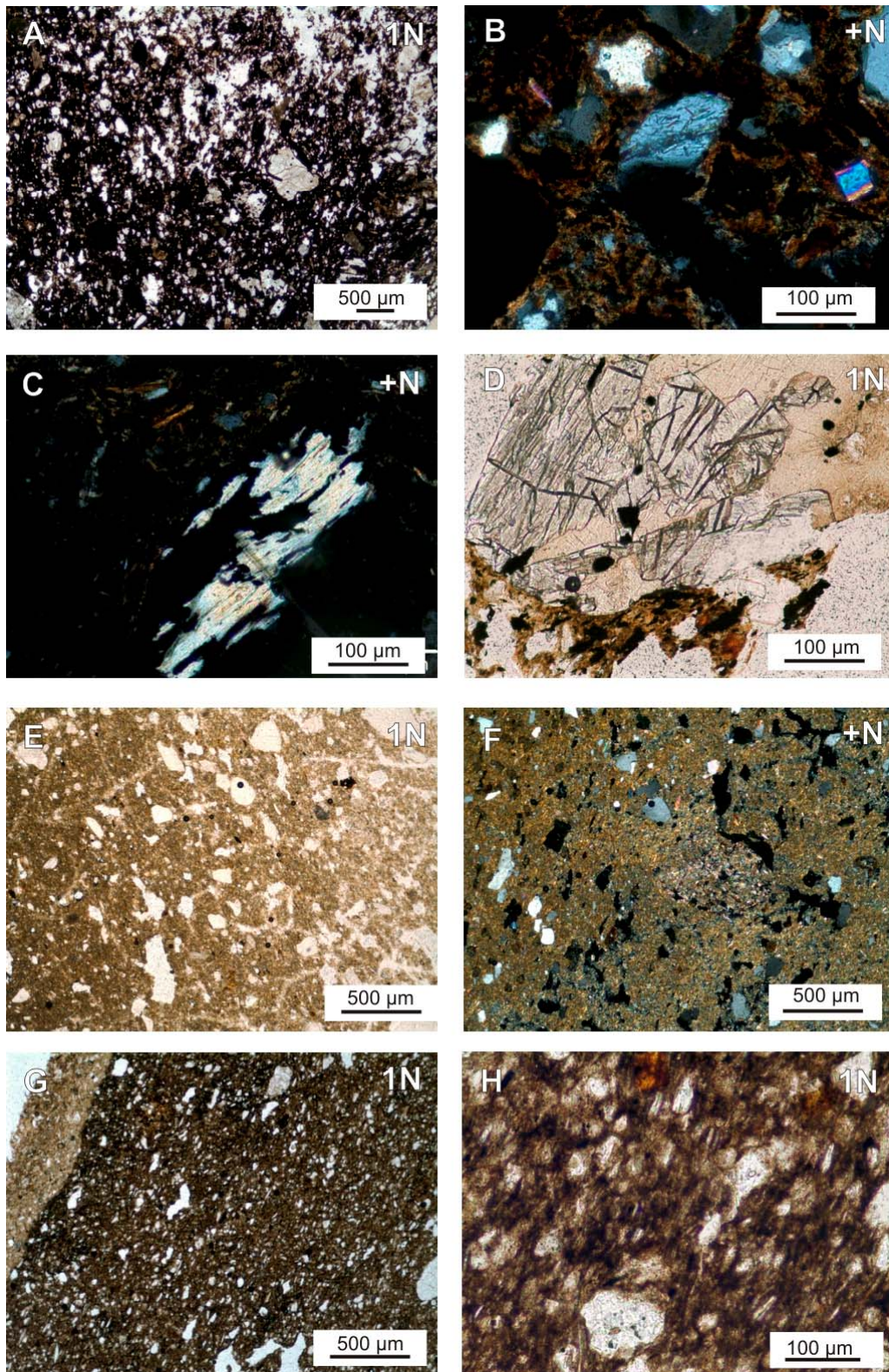
3. ábra Grafitos és nem grafitos kerámiák szöveti jellegzetességei (polarizációs mikroszkópi felvételek). A. Grafitos kerámia szöve (Ltsz. 1.58597.19.11, 1N), B. Grafitos kerámiában földpát által bezárt cirkon- és apatitzárványok, mellette turmalin és kvarc (Ltsz. 1.58597.6.6, +N), C. Grafitos kerámiában sillimanit (Ltsz. 1.58597.120.2, +N), D. Grafitos kerámiában kianitos-grafitos közettörmelék (Ltsz. 1.58597.6.6, 1N), E és F. Nem grafitos kerámia szöve: barna alanyag, kvarc és földpát nem-plasztikus elegyrészek (Ltsz. 1.58597.157.1, 1N ill. +N), G. Nem grafitos, szendvicsszerkezetű kerámia világos szegéllyel és sötét maggal, kvarc, földpát és muszkovit nem-plasztikus elegyrészekkel (Ltsz. 1.58597.120.10, 1N), H. Nem grafitos kerámiában cirkon- és apatitzárvány földpátban (Ltsz. 1.58597.35.7, 1N).
