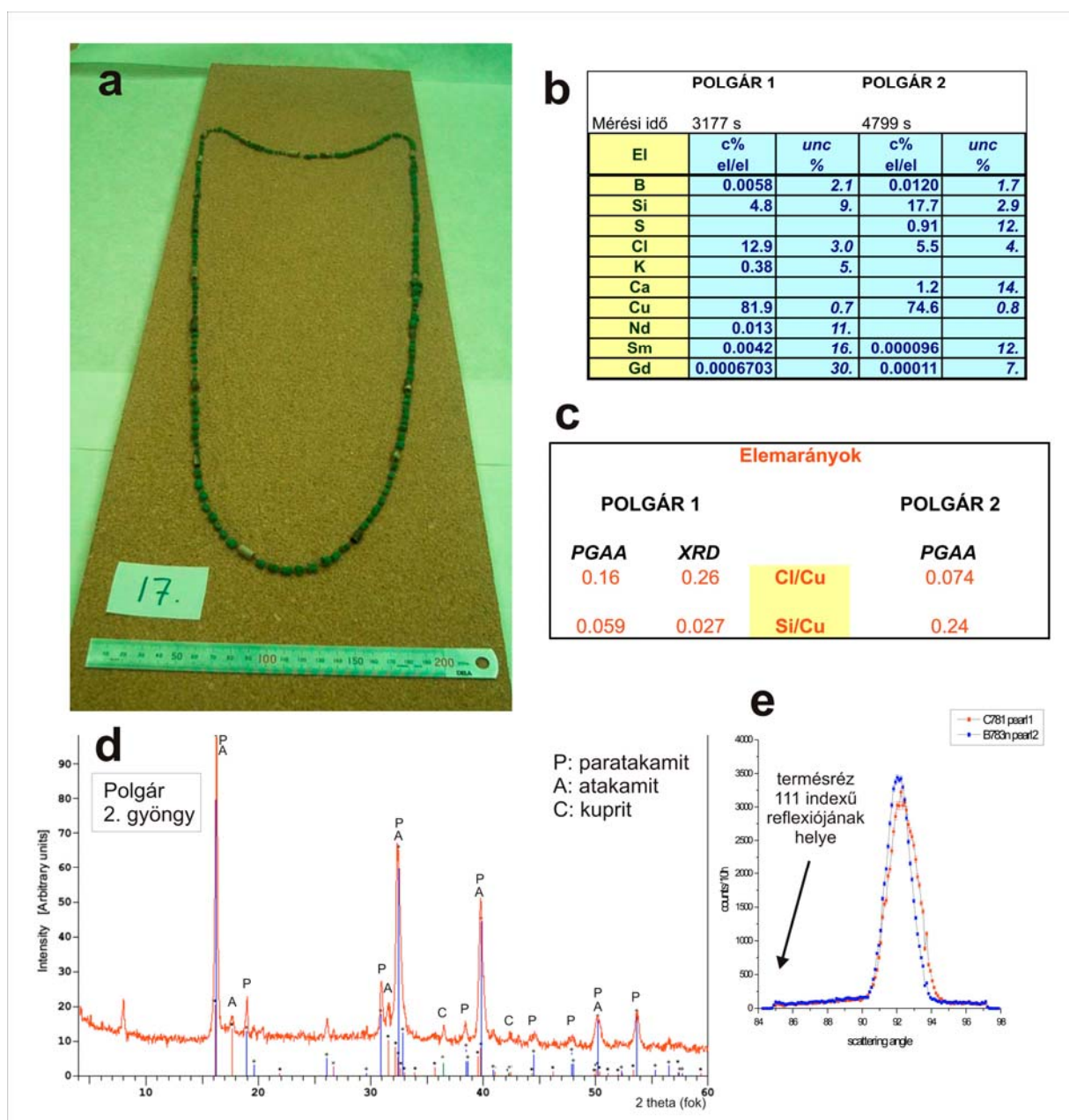
1. ábra: A Polgár-Csőszhalom neolitik lelőhelyről előkerült (a) gyöngysor két, eredetileg réz anyagú gyöngyszemének (b) kémiai összetétele PGAA vizsgálatok alapján, (c) kalkulált Cl/Cu és Si/Cu arányai, (d) a 2. gyöngy felületi fázisösszetétele röntgendiffrakciós vizsgálatok alapján, illetve (e) a gyöngyök átlagos ásványos összetétele neutron diffrakciós vizsgálatok alapján.
