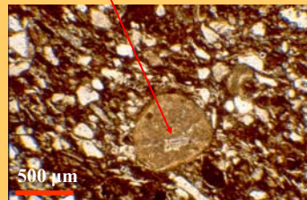
Kovaszivacstű mészkőben
