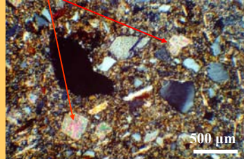
Elsődleges kalcit
