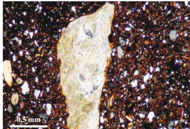
5. kép Talkpala törmelék vaskori kerámiában (Vaskeresztes) [+ Nikol]
