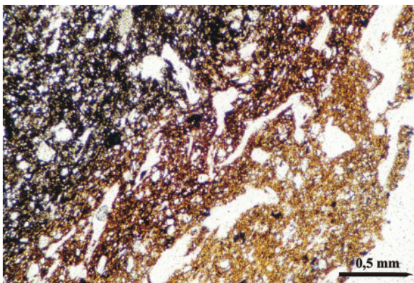
23. kép A kiégetés és hűntartás során az oxidációs-redukációs viszonyok változása miatt kialakuló szegély mikroszkópi képe, neolitikus kerámiában (Körös kultúra, Szarvas) [1 Nikol]
